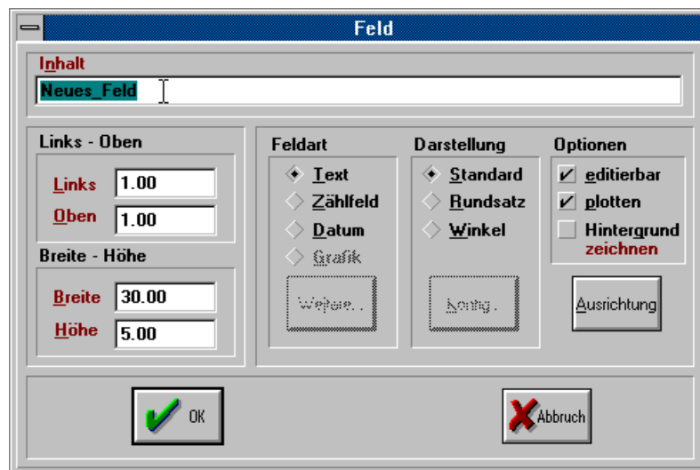
Abbildung 8: Der Felddialog - Position, Größe, Feldart und weitere Einstellungen
