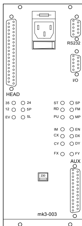
Vorderansicht der Steuerung
