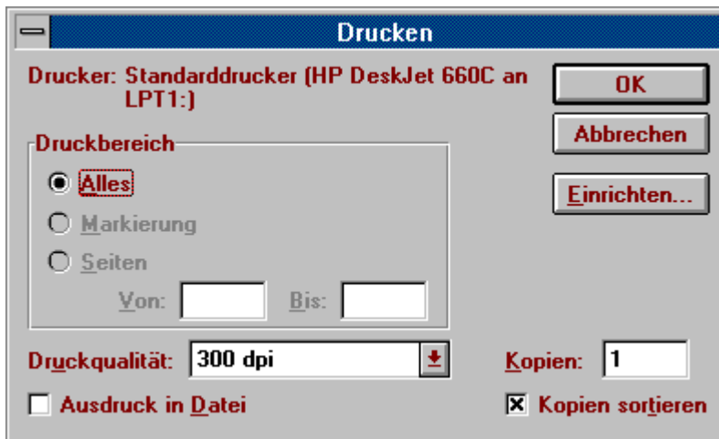
Abbildung 22: Dialog Drucken
