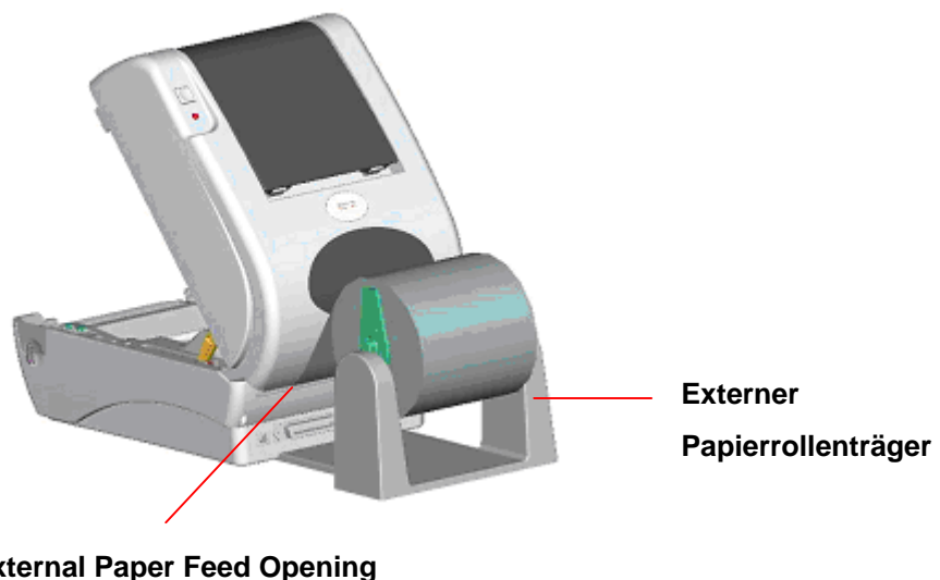
Abb. 10 Installation des externen Etikettenrollenträgers (I)
