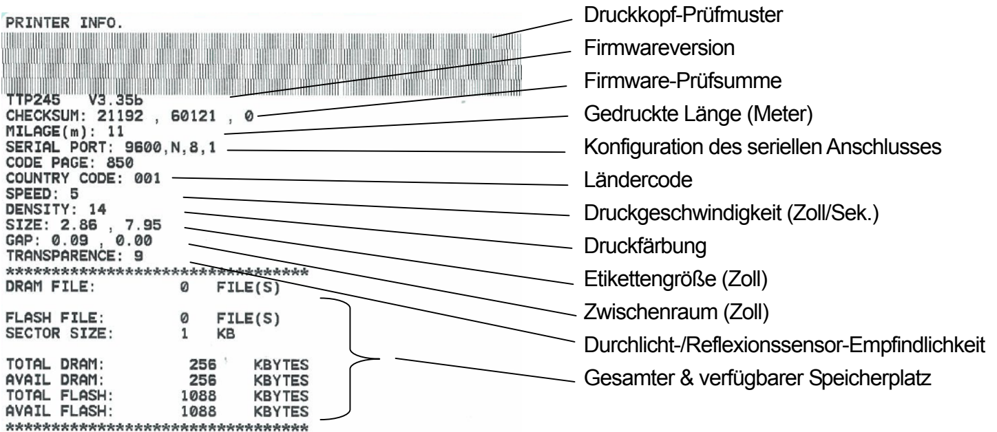
Abb. 29 Selbsttest-Ausdruck
