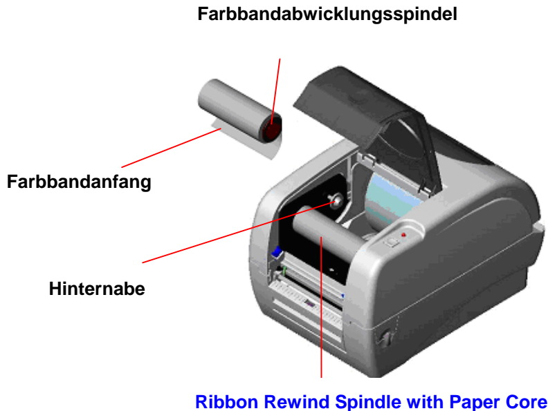
Abb. 5 Farbbandinstallation (II)
