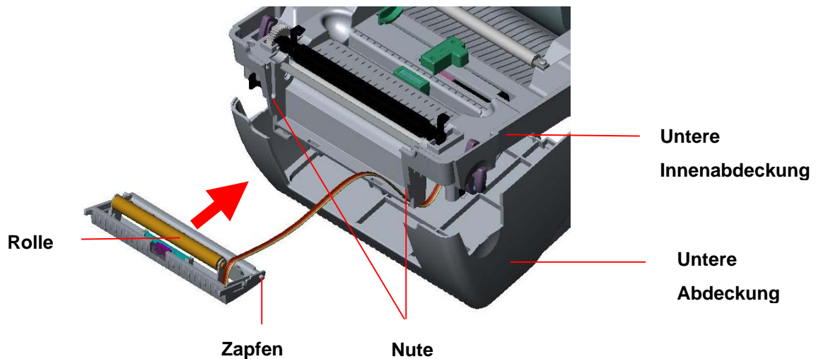
Abb. 16 Spendeeinrichtungsinstallation (I)
