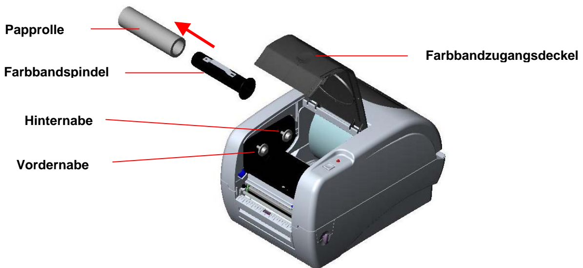
Abb. 4 Farbbandinstallation (I)
