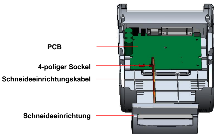
Abb. 24 Schneideeinrichtungsinstallation
